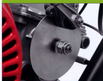
Freno a disco sincronizzato con comando frizione Disc brake synchronized with clutch lever
